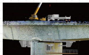
▲ 3D で作成した施工手順のイメージ
