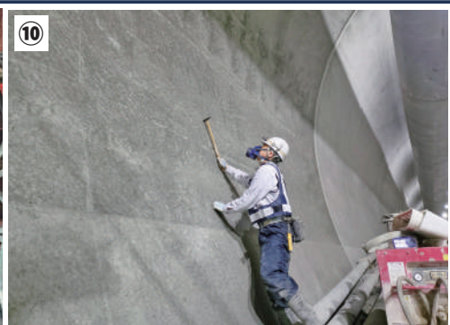
⑨ セントルの点検と、覆工後のコンクリートの表面をハンマーでたたき、空洞などがないか打音検査⑩を行う吉田主任。技術者の経験と感性・技術力が活きる場面。
